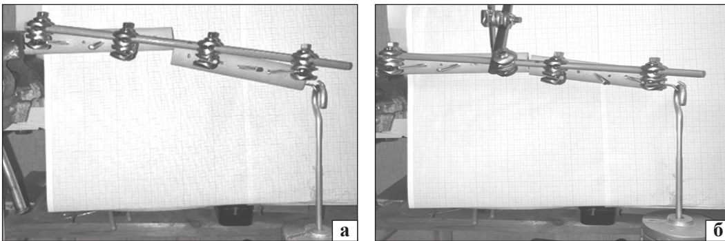
Рис. 8. Величина переміщення дистального «уламка» за максимального навантаження моделі зі застосуванням апарата «Orthofix» за умов розташування усіх стрижнів у фронтальній площині (а) і під час заведення одного стрижня, що в проксимальному уламку в площині, яка під 45^\circ до фронтальної (б) (параметри конструкції 9, 14 в таблиці 1)
