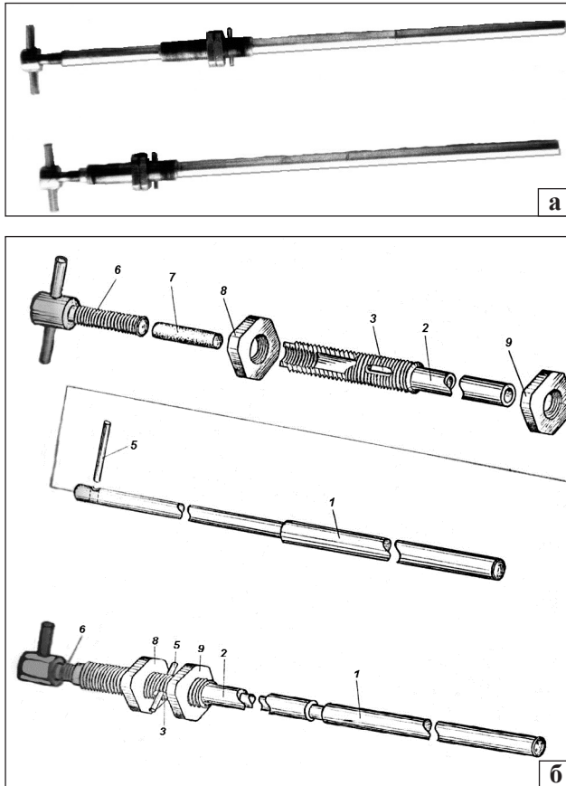
Рис. 3. Внешний вид (а) и схема (б) наружной опоры стержневого аппарата с регулируемым демпфером
