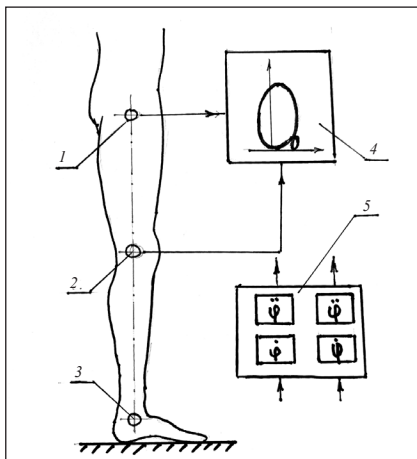
Рис. 2. Схема реєстрації біомеханічних патернів рухів: 1, 2, 3 — гоніометри на кульшовому, колінному та над'яtkово-гомілковому суглобах; 4 — двокоординатний реєстратор; 5 — блок диференціювання
