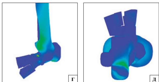
Рис. 3. Картина розподілу напружень у моделі стопи з коригувальним гвинтом у п'ятковій кістці: загальний вигляд із медіального боку (а), із медіального без надп'яtkової кістки та імплантата (б), із латерального без надп'яtkової кістки та імплантата (в), опорна поверхня (г), опорна поверхня (д)
