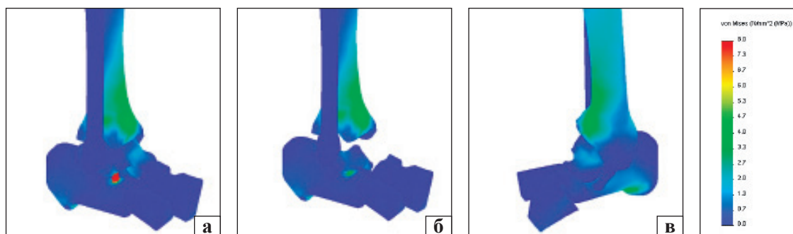
Рис. 3. Картина розподілу напружень у моделі стопи з коригувальним гвинтом у п'ятковій кістці: загальний вигляд із медіального боку (а), із медіального без надп'яtkової кістки та імплантата (б), із латерального без надп'яtkової кістки та імплантата (в), опорна поверхня (г), опорна поверхня (д)
