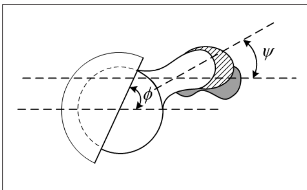
Рис. 7. Схема встановлення ендопротеза кульшового суглоба: \phi — кут антеверсії чашки, \psi — кут антеторсії ніжки
